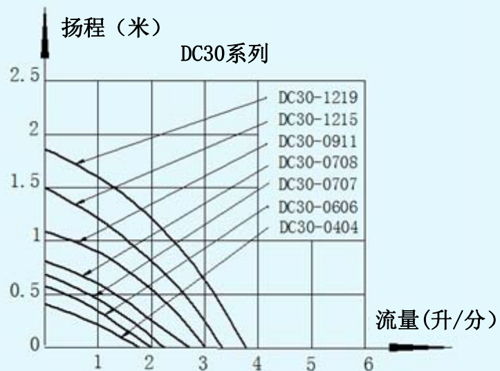
扬程-流量曲线图
