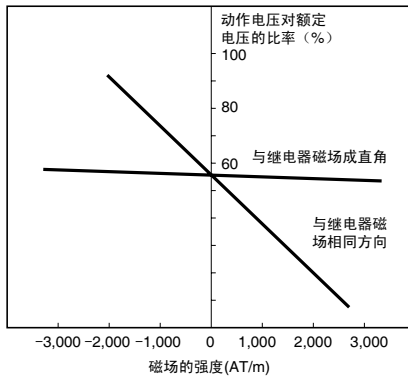
外部磁场方向与导线继电器的动作特性 LA1 的场合
