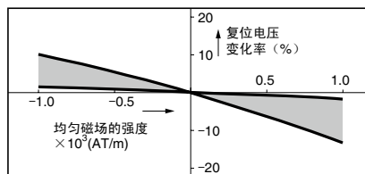
外部均匀磁场下的磁干扰试验(2) LA1 的场合
