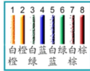
T568B
