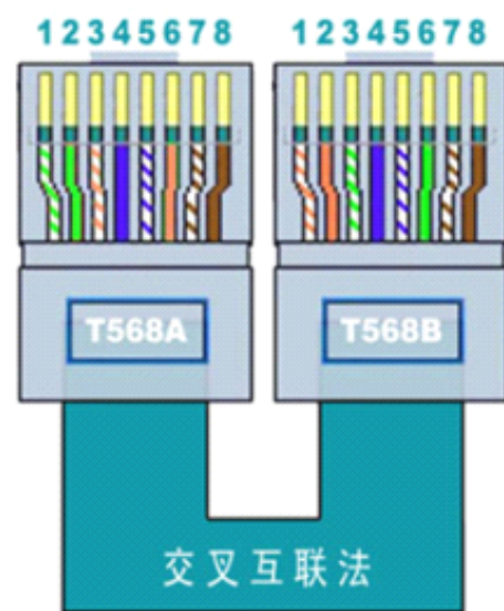
T568B
