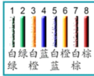
T568A
