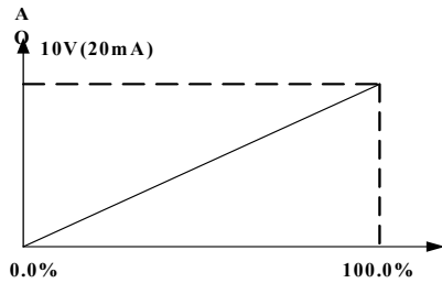
图6-13 给定量与模拟输出对应关系
