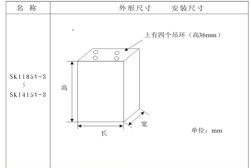
图 1-4 变频器 185 以上外形尺寸图
