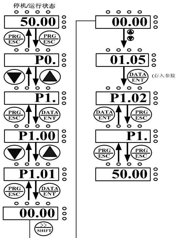
图5-2 三级菜单操作流程
