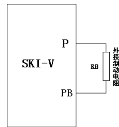
图 1-4 制动电阻的安装
