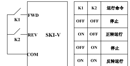
图 6-9 两线式控制 (使能与方向分离)
