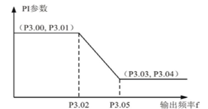
图6-5 PI参数示意图
