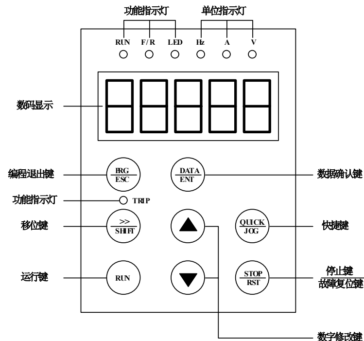
图 5-1 操作面板示意图
