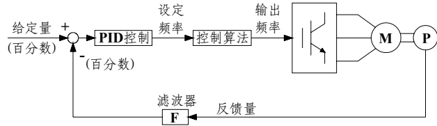
图6-18 过程PID原理框图
