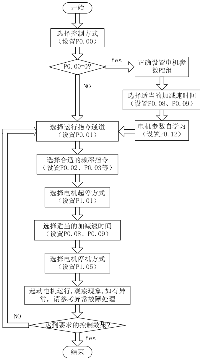
图 5-3 快速调试流程图
