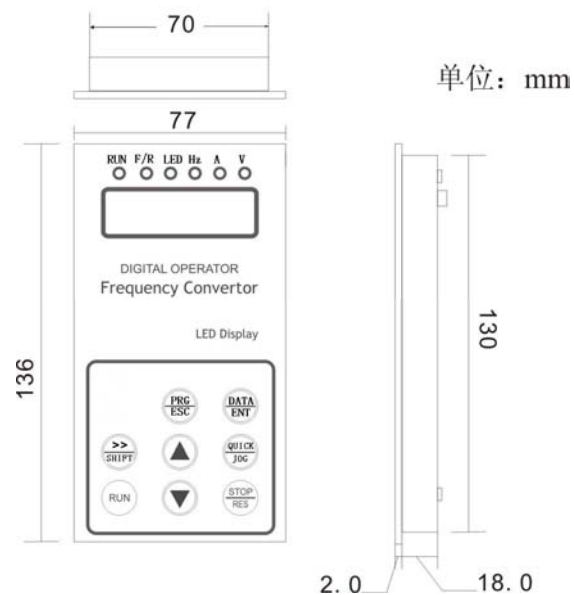
图 1-6 变频器操作面板尺寸 (大): SKI-7D5V-3000~SKI-415V-3000
