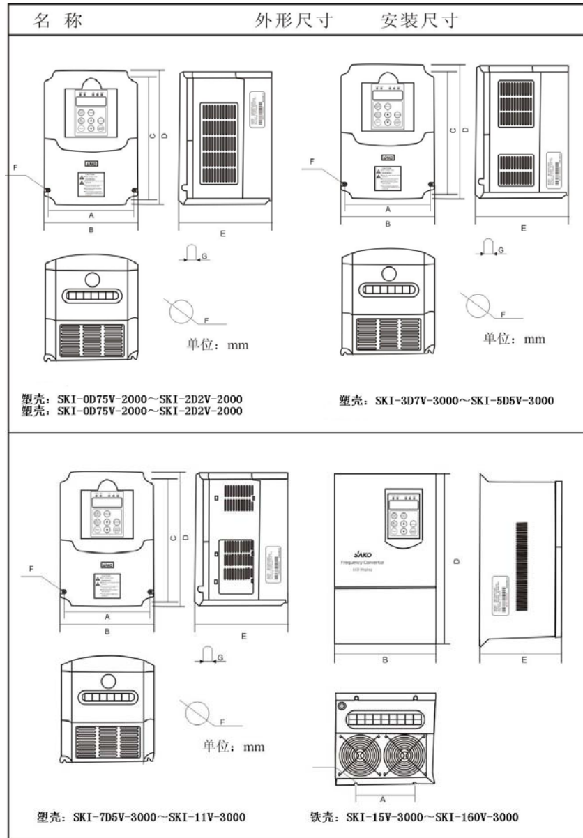
图 1-3 变频器 160KW 以下外形尺寸图
