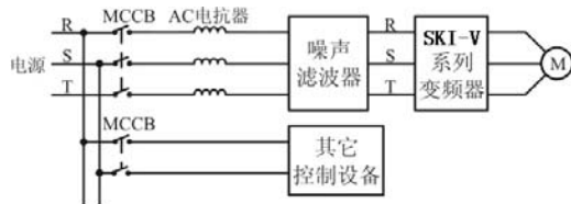
图 4-15 主回路电源侧连接图
