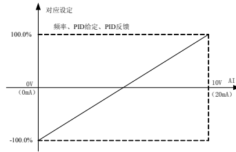
图6-12 模拟给定与设定量的对应关系
