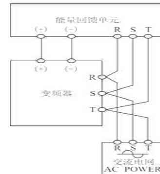
图 4-17 能量回馈单元连接图
