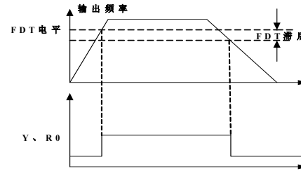
图6-16 FDT电平示意图
