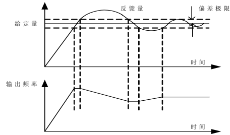
图6-19 偏差极限与输出频率的对应关系
