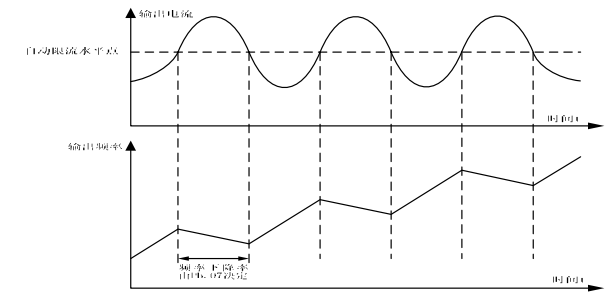
图6-23 过流失速功能
