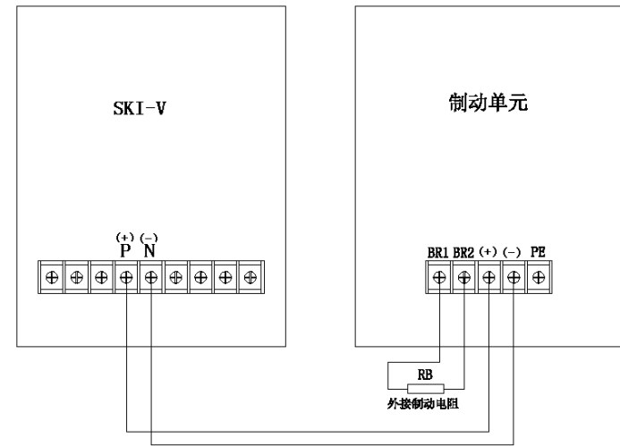
图 1-5 制动单元的连接
