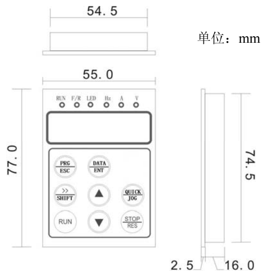
图 1-5 变频器操作面板尺寸 (小): SKI-0D75V-2000~SKI-5D5V-2000 SKI-0D75V-3000~SKI-5D5V-3000
