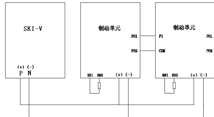
图 1-6 制动单元的并联连接
