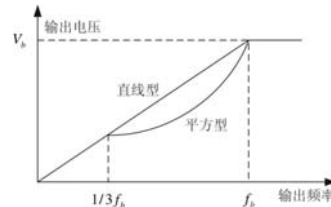
图6-6 V/F曲线示意图
