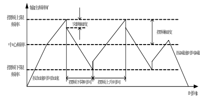
图6-15 摆频运行示意图
