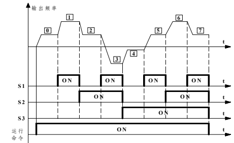
图6-20 多段速度运行逻辑图
