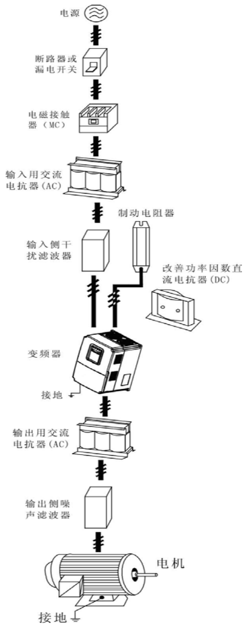
图 4-1 外围设备的连接图
