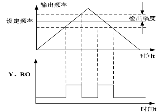
图6-17 频率到达检出幅值示意图
