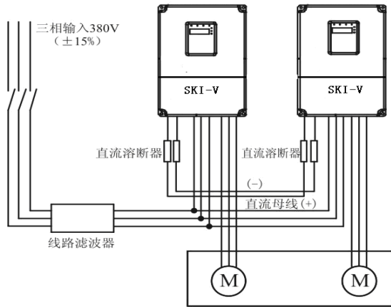
图 4-18 共直流母线的连接
