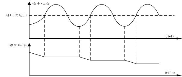
图6-22 过压失速功能
