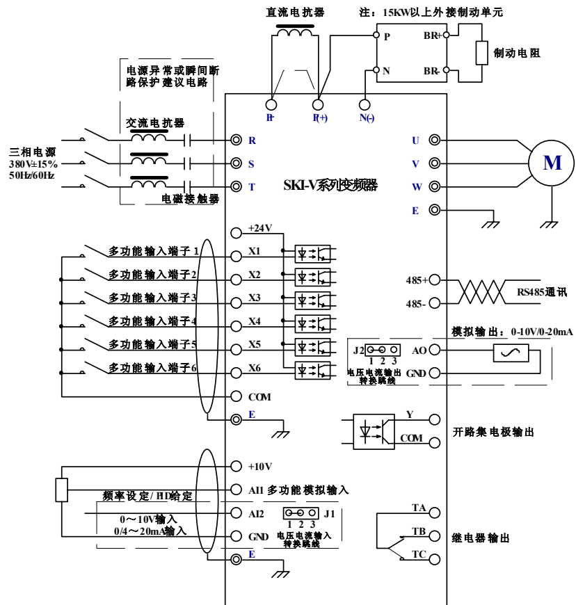
图 4-2 标准接线图
