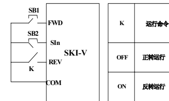
图 6-10 三线式控制模式 1
