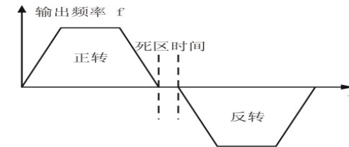
图6-4 正反转死区时间示意图
