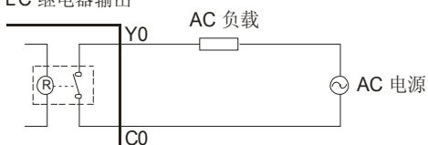
PLC 继电器输出
