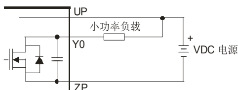
PLC 晶体管输出
