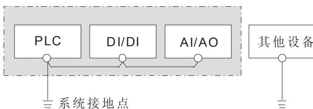
第三种接地(接地阻抗 100\Omega 以下)
