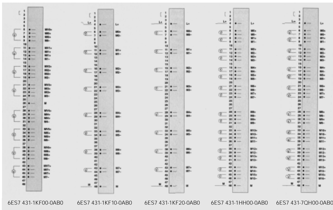
图 19 用于电压测量的模拟量输入模板的端子接线图
