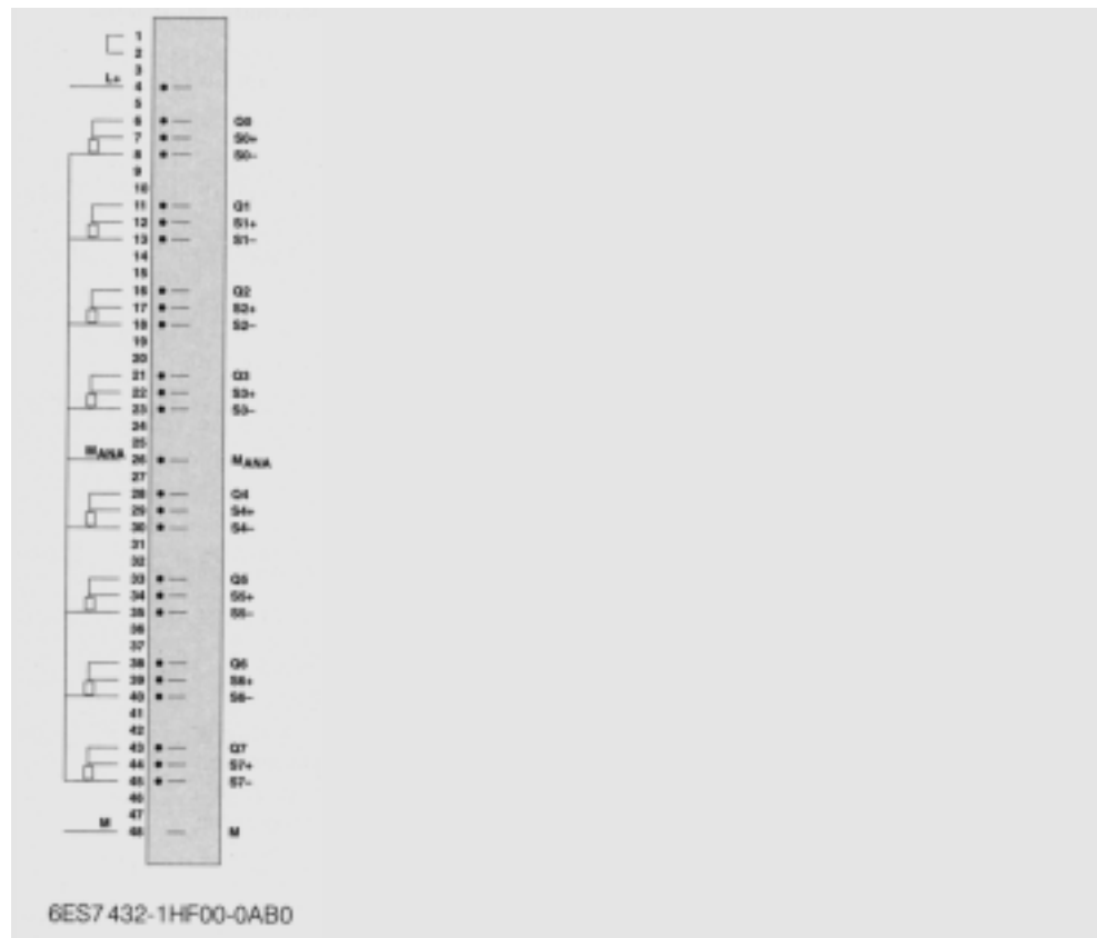
图 20 模拟量输出模板的端子接线图
