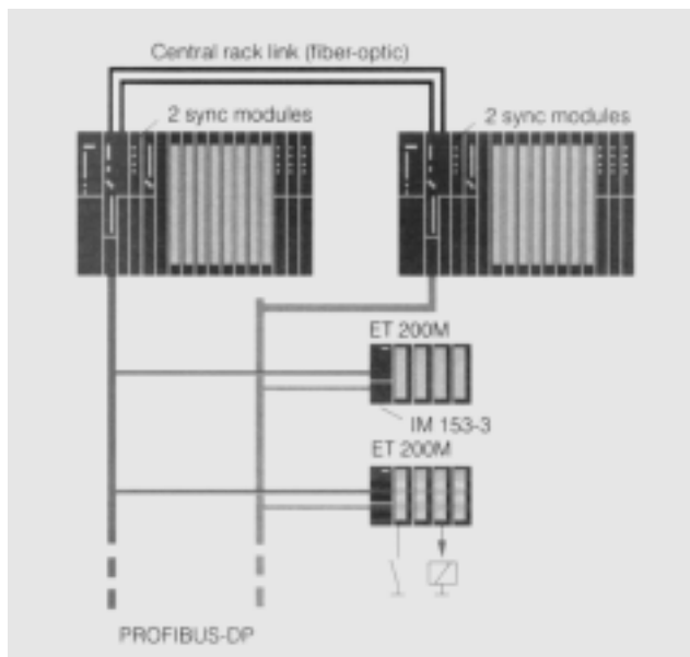
图 10 切换式配置
