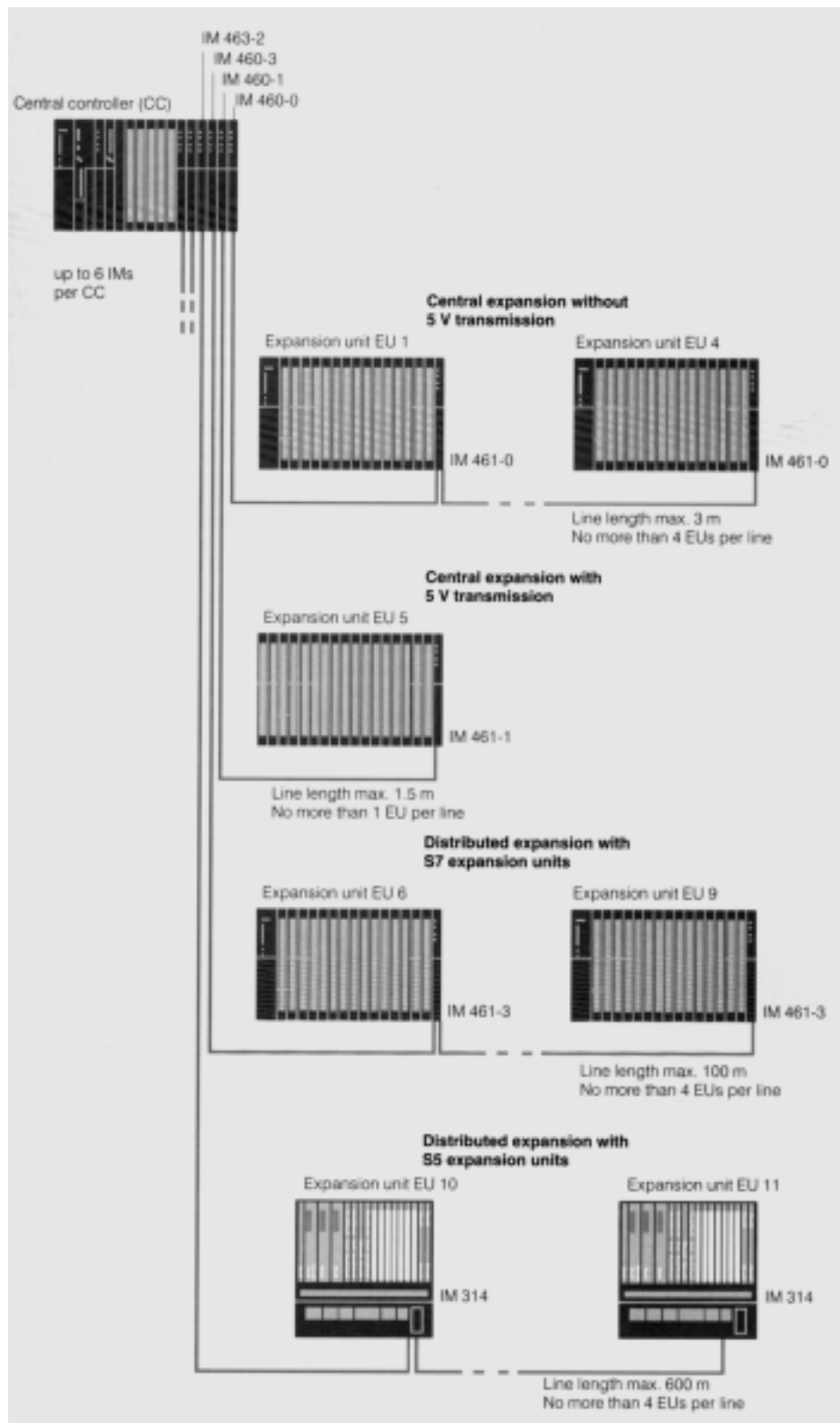
图 3 S7-400 可能的扩展型式
