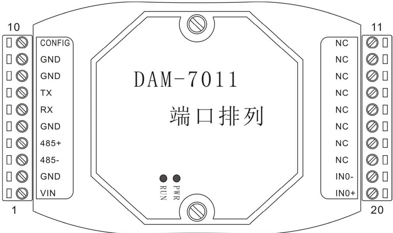
图 4-1 DAM-7011 模块端口位置示意图
