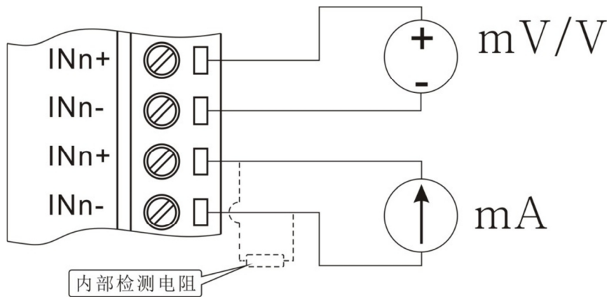
图 3-1 DAM-70X1 模拟量输入接线示意图
