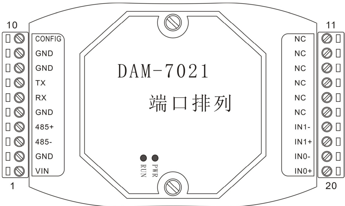
图 4-2 DAM-7021 模块端口位置示意图
