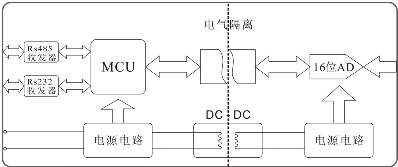
图 1-2 DAM-70X1 工作原理框图
