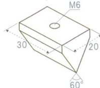
くさび圧子 ジュラコン製
