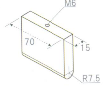
半円柱圧子 ジュラコン製 CJ-SC7015
