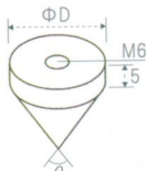
円錐圧子 ジュラコン製 CJ-C[θ]-[D]
