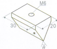
くさび圧子 ジュラコン製 CJ-W[θ]-30
