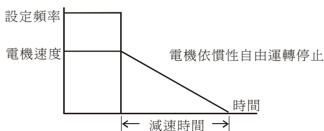
運轉指令 ON OFF 圖二：自由運轉
