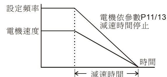
運轉指令 ON OFF 圖一：減速煞車
