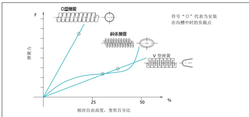
弹簧负载曲线图
