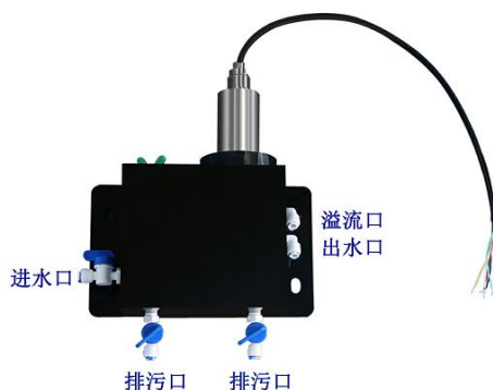
图三：流通式安装
