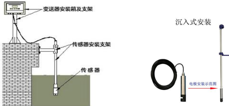
图二 TSS 传感器安装示意图
