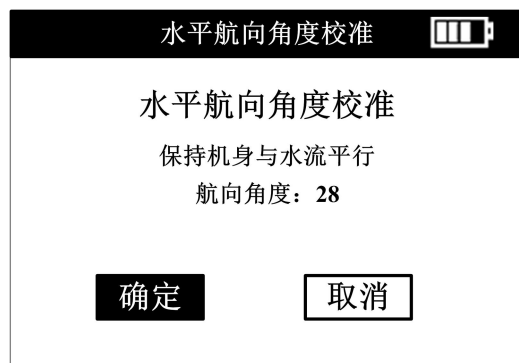
图 18 航向角度校准
