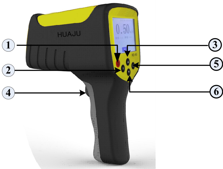
图 2 按键功能介绍
