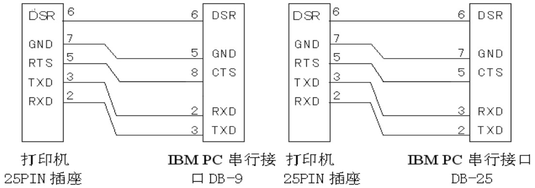
图 3-17 DB25 孔型串行接口与 PC 机串行口连接示意图
