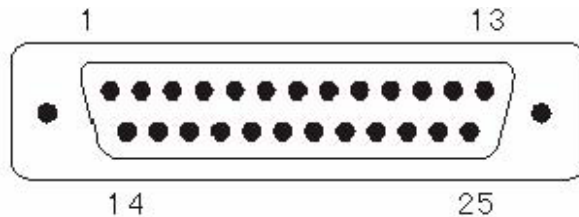
图3-19 DB25针型并行接口插座引脚序号
